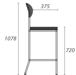
PS44HCH-72 高腳椅, 座深 37.5 公分
