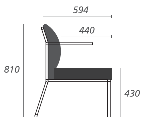
PS57SL 斜背沙發椅, 座深 44 公分
