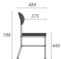
PS44CH-44 餐椅, 座深 37.5 公分
